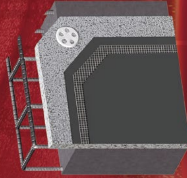
现浇混凝土保温外墙系统 【保温模板（硅塑保温板）】
